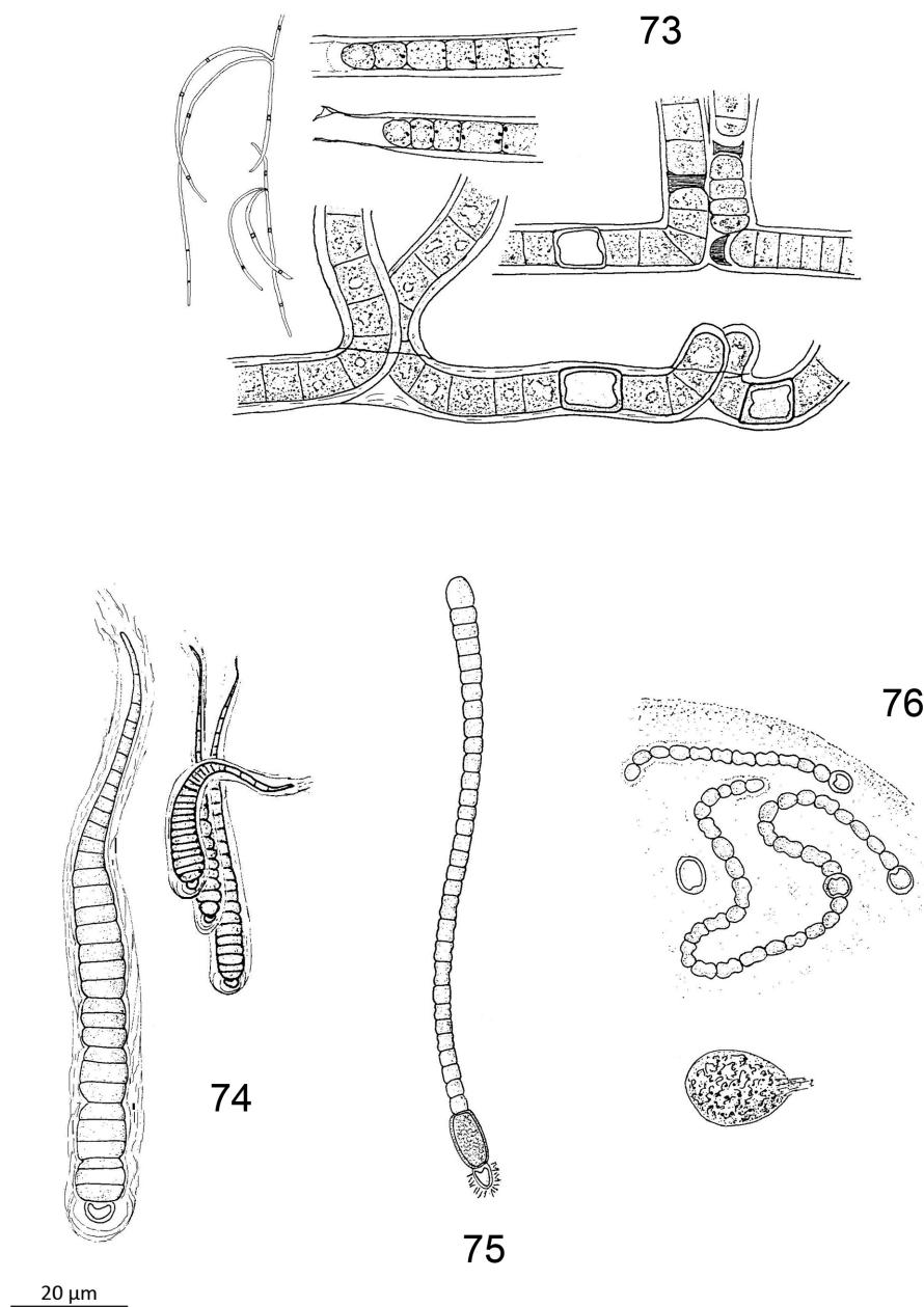
Figs. 73-76. Cyanoprokaryota. Nostocales. 73. Scytonema bohneri (talo, ramificaciones y ápices) 74. Calothrix parietina (filamento y talo) 75. Cyindrospermum stagnale . 76. Nostoc muscorum (filamento y colonia de 2 mm).
