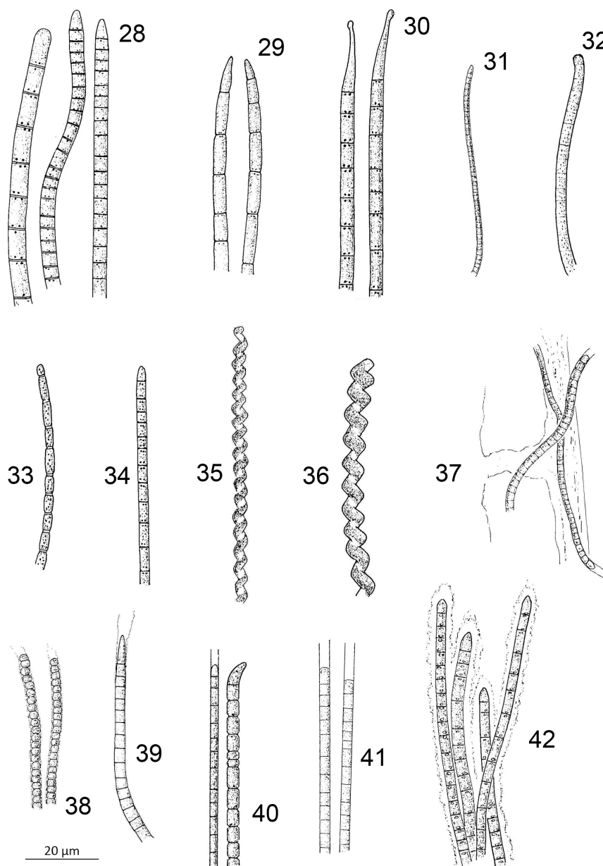
Figs. 28-42. Cyanoprokaryota. Oscillatoriales. 28. Geitlerinema amphibium . 29. G. claricentrosom . 30. G. splendidum . 31. Jaaginema angustissimum . 32. J. geitleri . 33. J. geminatum . 34. J. quadripunctulatum . 35. Spirulina major . 36. S. nordstedtii . 37. Leibleinia epiphytica . 38. Leptolyngbya foveolarum . 39. L. laminosa . 40. L. tenuis . 41. L. valderiana . 42. Schizotrrix lardacea .
