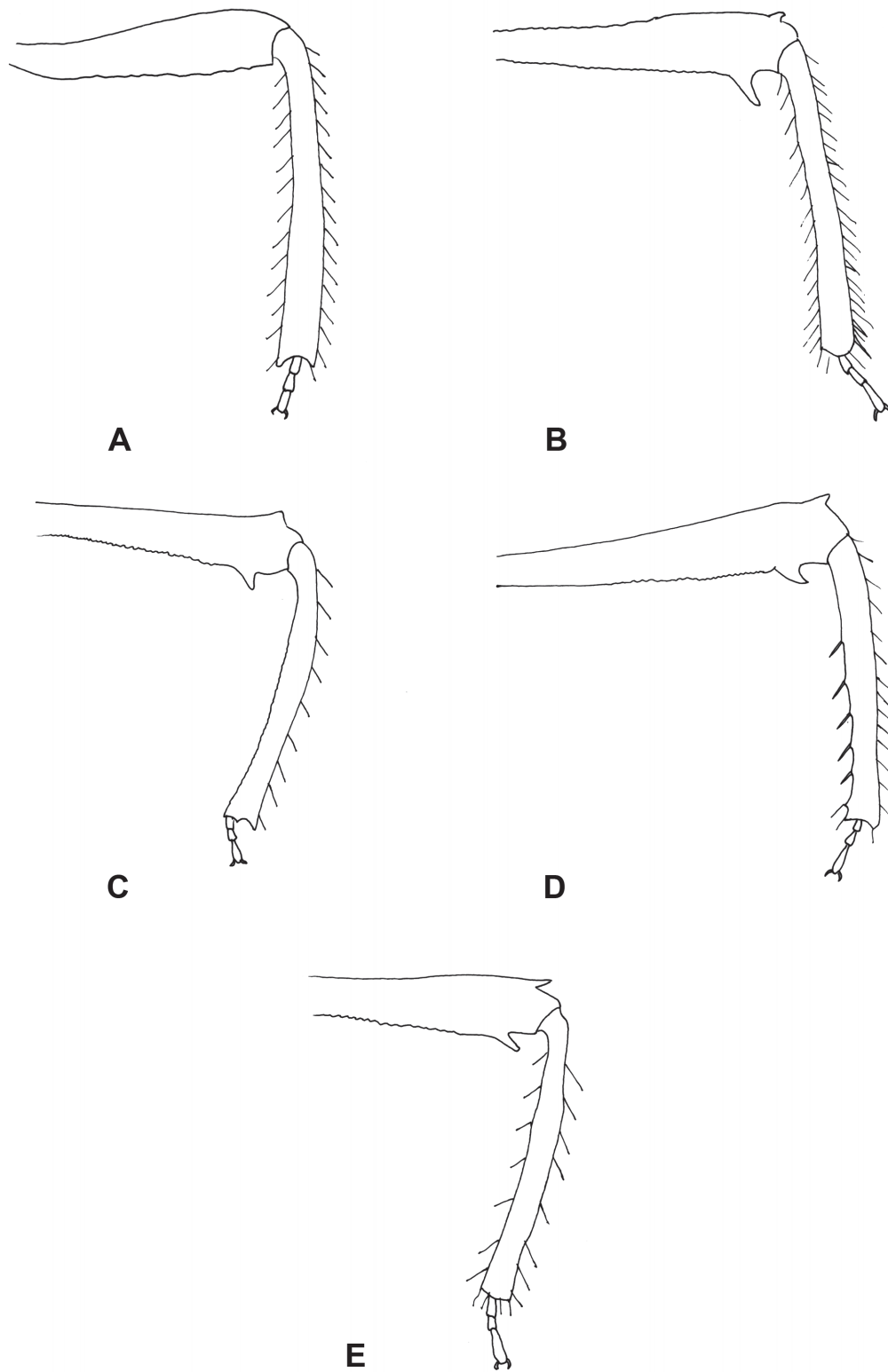
Figura 5. Fémur posterior del macho de las especies de Lattinestus . A, L. amplius ; B, L. barrera ; C, L. branstetteri ; D, L. cervantes ; E, L. egeri .
