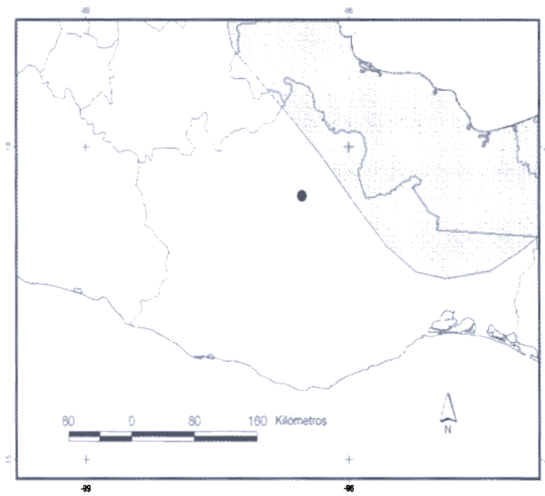
Figura 2. Mapa de distribución conocida de A. paca (Villa y Cervantes, 2003). La marca indica las localidades donde se registró la especie.
